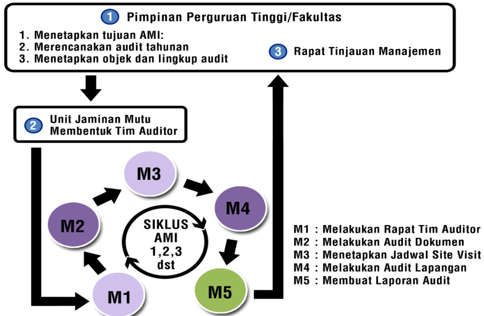
Gambar 3.1 Siklus Audit
